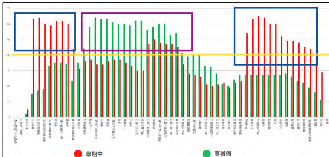
圖10 往豐原晚尖峰學期中及寒暑假車上人數比較
