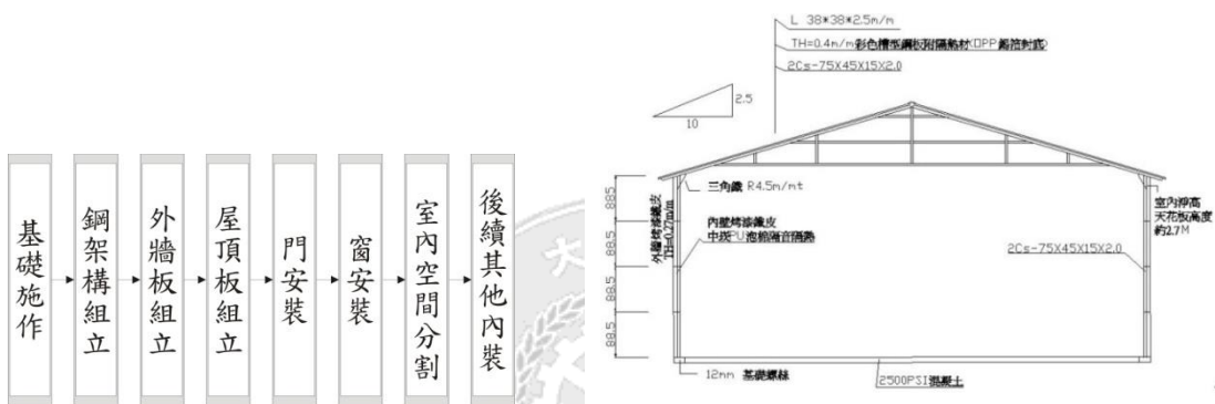
圖 2、組合屋施工流程圖
