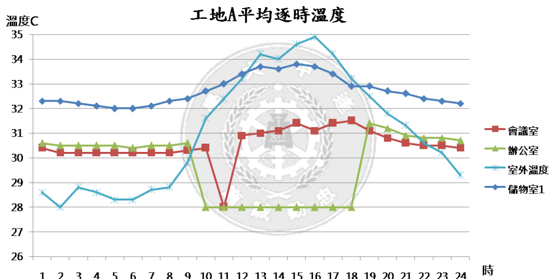
圖 11、工地 A 平均逐時溫度
