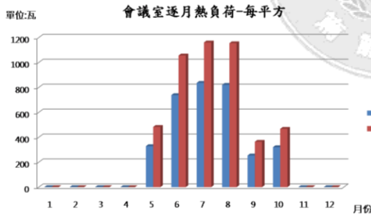
圖 7、會議室逐月每平方熱負荷圖
