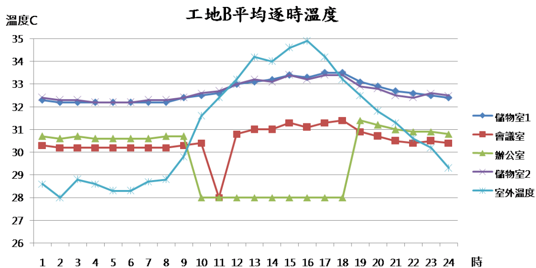
圖 12、工地 B 平均逐時溫度
