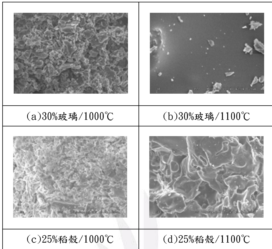
圖 4-12 燒結試體之 SEM 圖(×2000)
